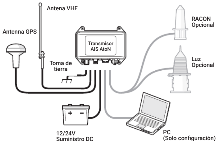
ESQUEMA GENERAL DE CONEXIÓN BALIZA A UNIDAD AIS MTA.
